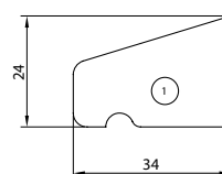
LISTELLO DEL GOCCIOLATOIO 1 STANDARD
