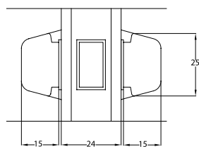
INGLESINA VIENNESE VERTICALE 25 mm
