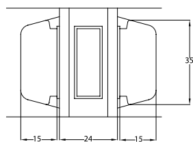
INGLESINA VIENNESE VERTICALE 35 mm
