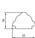
INGLESINA RETRO VERTICALE E ORIZZONTALE
